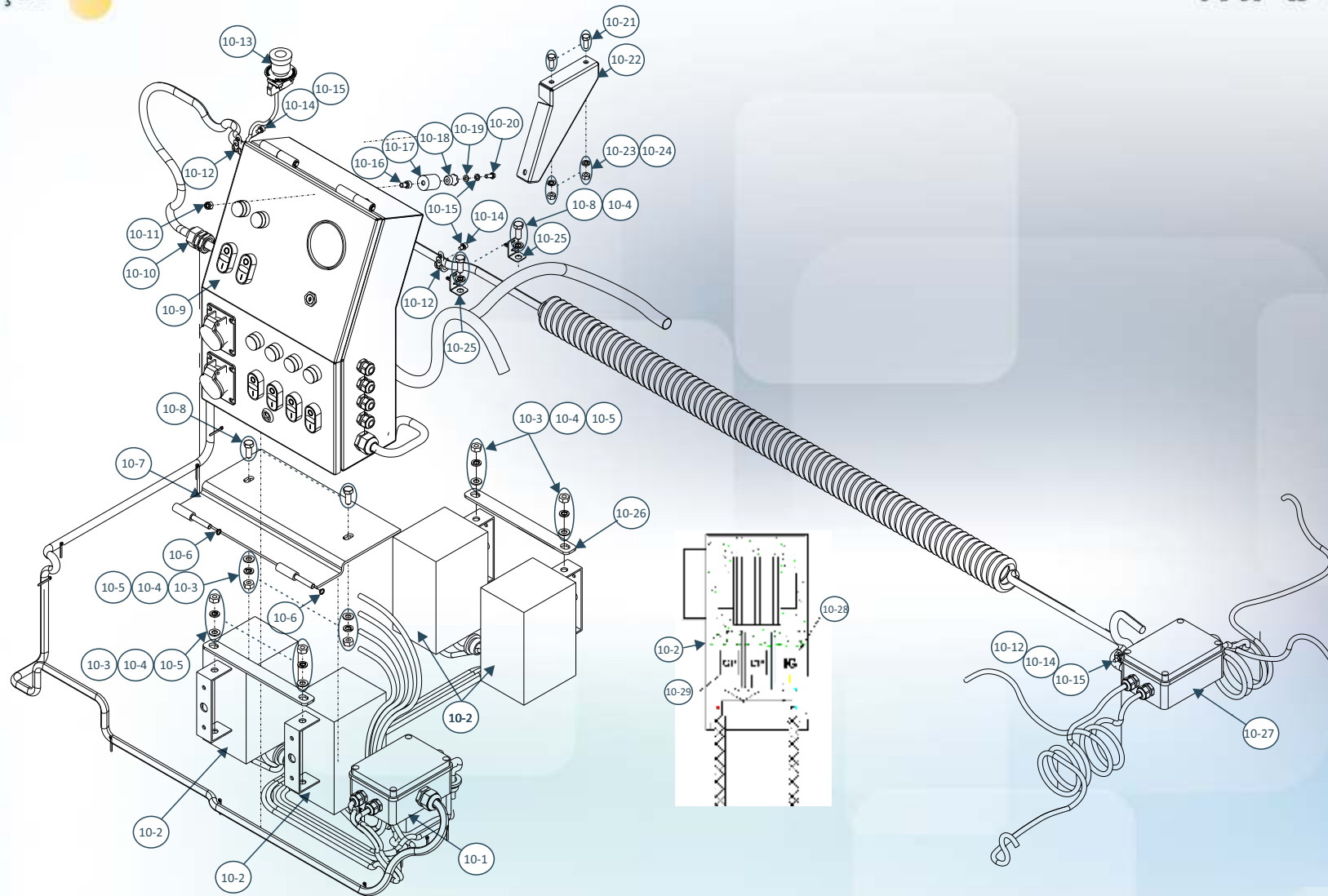
Montagem do Sistema Elétrico Parte 2 (Ligação dos reatores + Painei Elétrico) | 10-1 a 10-27
