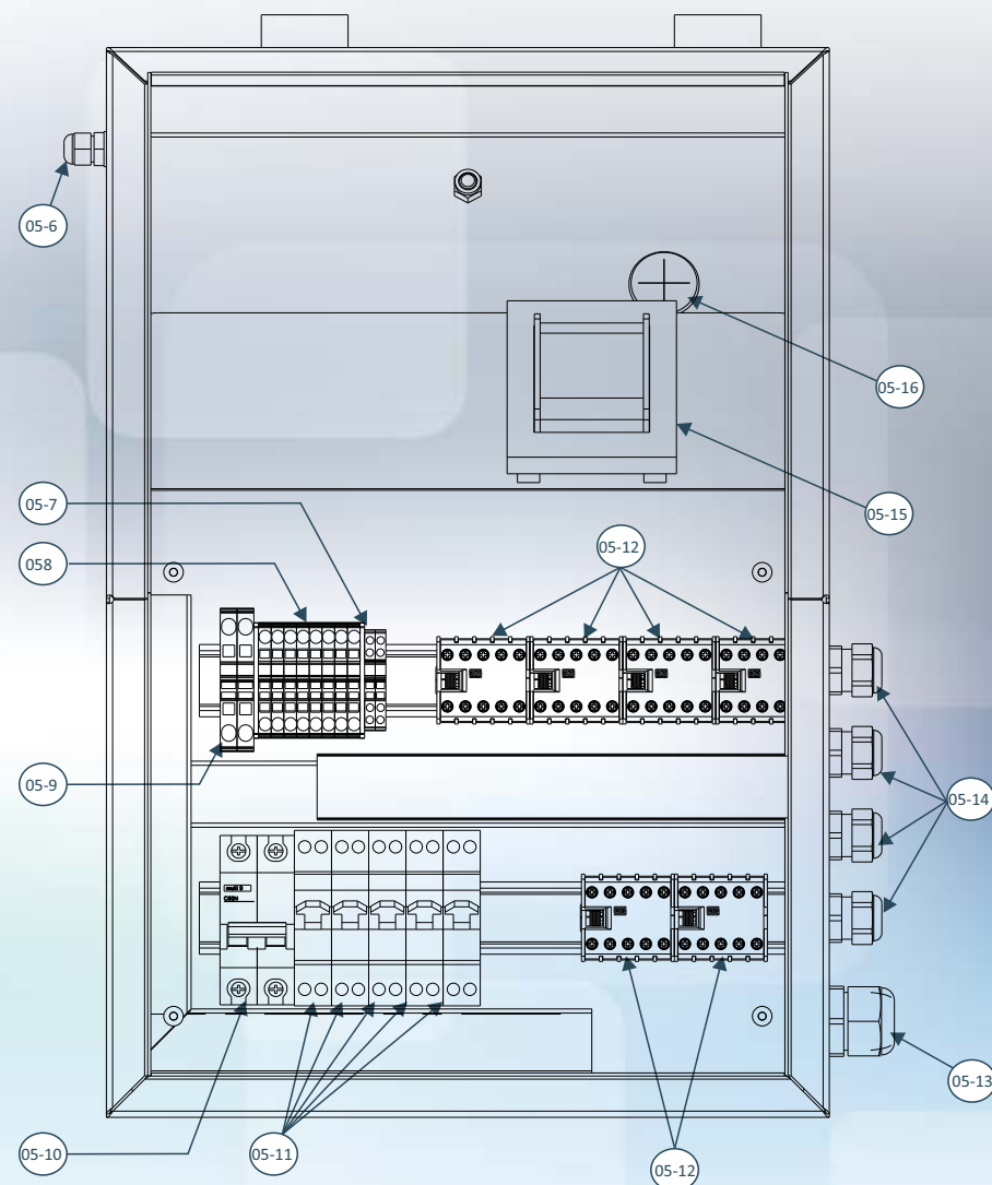
Montagem do Painel Elétrico (parte interna) | 05-6 a 05-16
