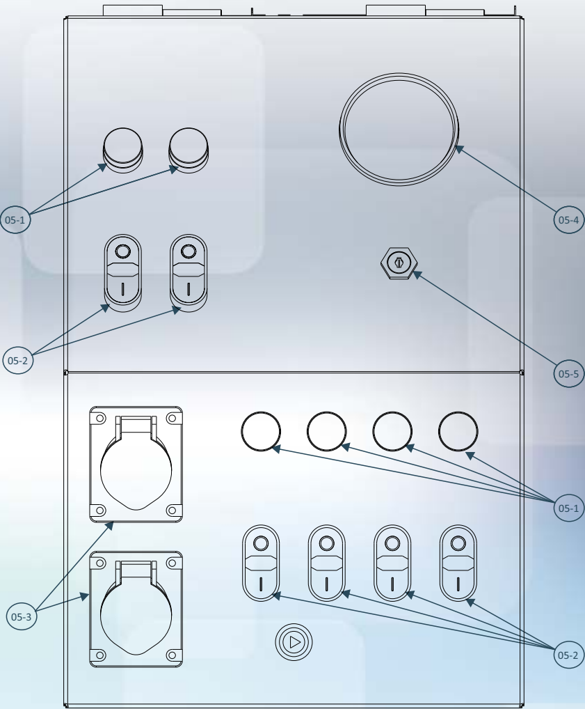
Montagem do Painei Elétrico (parte externa) | 05-1 a 05-5
