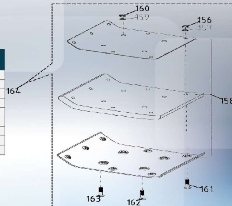
Conjunto Sapata | 156 a 164
