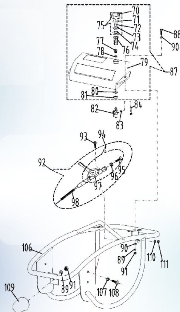
Conjunto Guidão de Operação e Tanque de Combustível | 70 a 111
