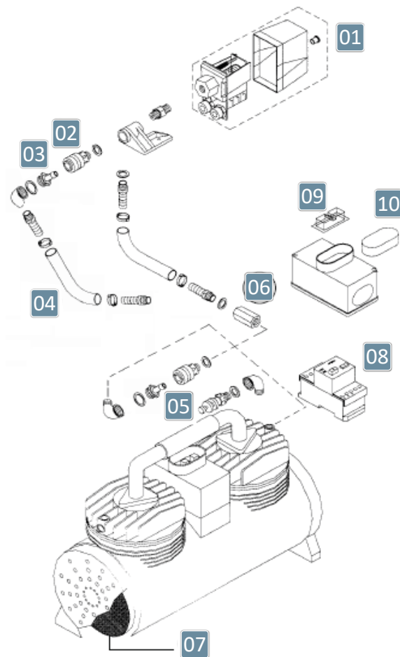
FIGURA 06 - CONJUNTO COMPRESSOR
