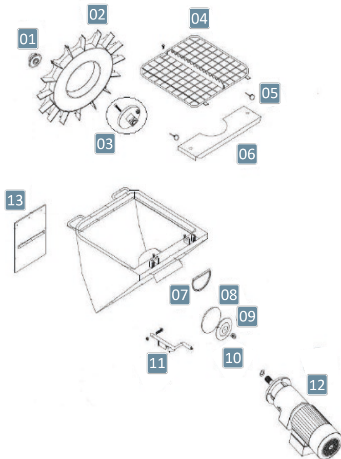
FIGURA 03 - TREMONHA
