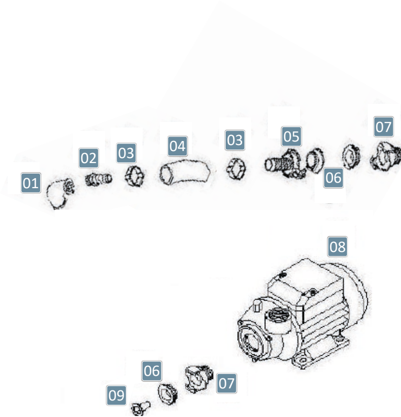
FIGURA 05 - CONJUNTO BOMBA DE ÁGUA
