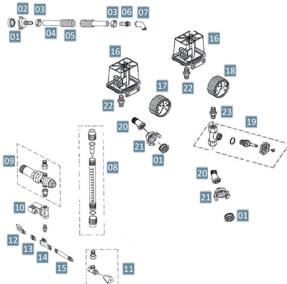
FIGURA 04 - GRUPO AR / ÁGUA
