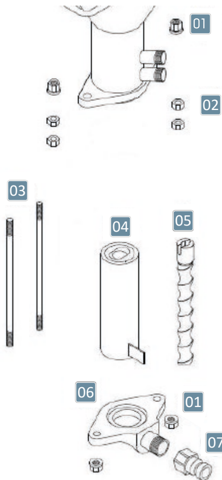
FIGURA 01 - SISTEMA BOMBA PARAFUSO
