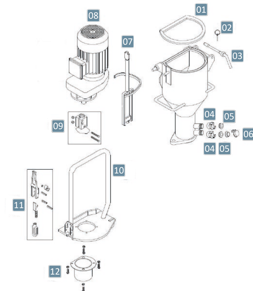
FIGURA 02 - CÂMARA MISTURADORA
