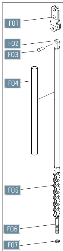
CONJUNTO VARILLA DE GATILLO
